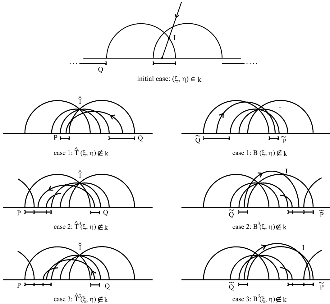
Fig. 9. Fundamental lemma.
