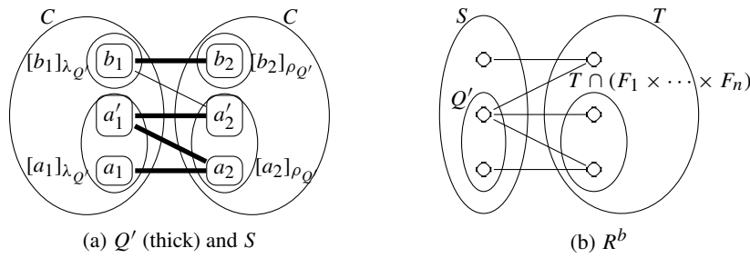
Fig. 6. The proof of Lemma 3.4.
