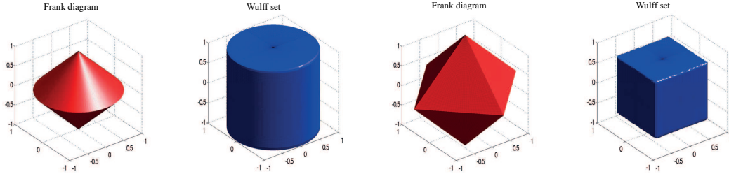
FIG. 5. Frank diagram and Wulff set: B_{\phi_4^o} , B_{\phi_4} , B_{\phi_5^o} , B_{\phi_5}
