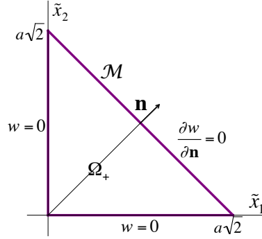
FIG. 5. Eigenvalue problem
