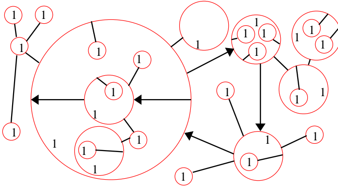
(d) Type- \delta configuration.
