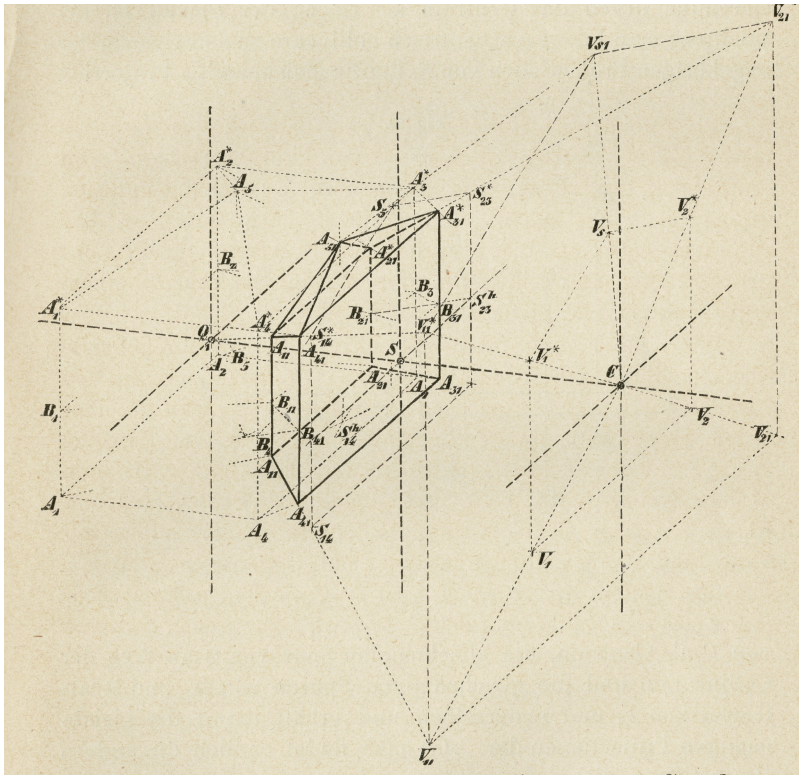
Abbildung 4 Modell eines Polyeders (Würfel mit aufgesetzter Pyramide, ganz links). Dessen Bild, das Modell, ist fett gedruckt. Bilder von Punkten sind durch den zusätzlichen Index 1 gekennzeichnet (z. B. ist A_{11} das Bild von Punkt A_1 ). (Fiedler 1871, 126)
