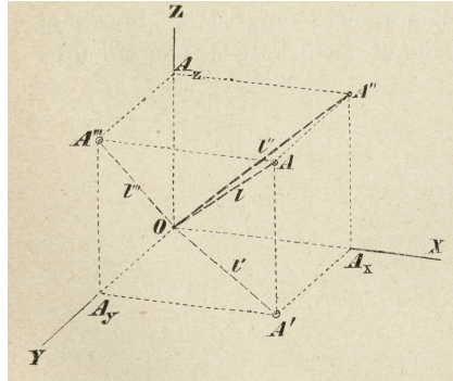
Abbildung 5. Punkt A mit seinen drei Projektionen (Fiedler 1871, 139)
