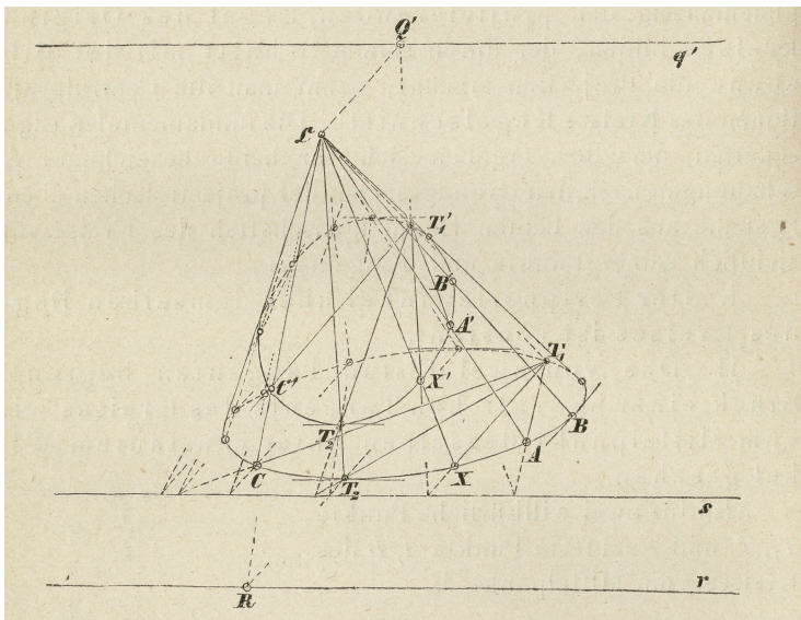
Abbildung 2. Kegelschnitt als Bild einer Zentralprojektion (Fiedler 1871, 72)
