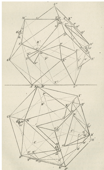
Abbildung 6. Durchdringung eines Ikosaeders mit einem Würfel (Fiedler 1871, 175)
