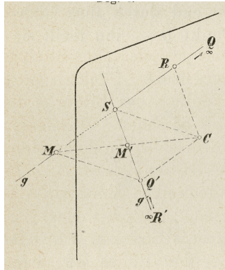
Abbildung 1. Fig. 4 aus Fiedler 1871, 9 2
