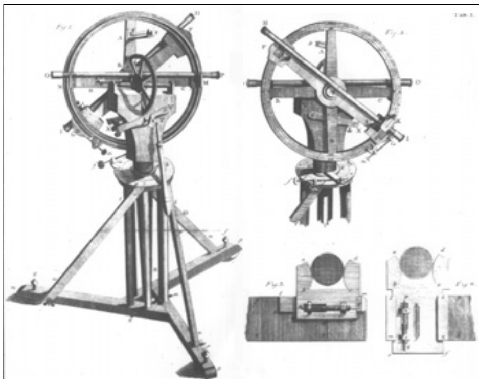
The geographical instrument shown in vertical position, from Thomas Bugge's Beskrivelse over den Opmaalings Maade som er brugt ved de Danske geografiske Kartter , København, 1779.
